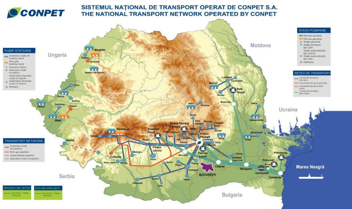
Grafic 17- Sistemul național de transport operat de CONPET
